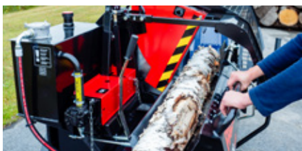
Einfache Stammverarbeitung dank eines stabilen Schneidetisches.
