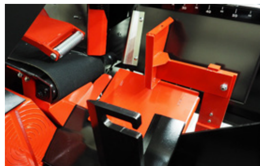
Die Fallplatte führt das Holz direkt in den Spaltschacht.
